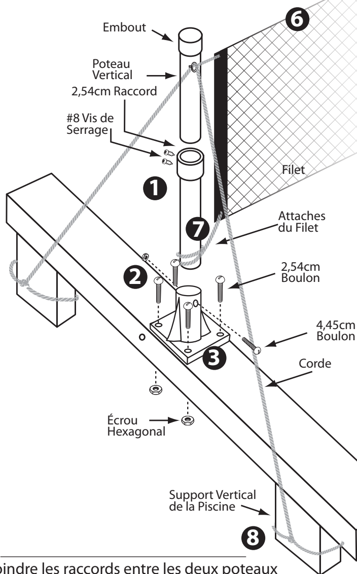
Détail du Poteau et de L'oeillet
